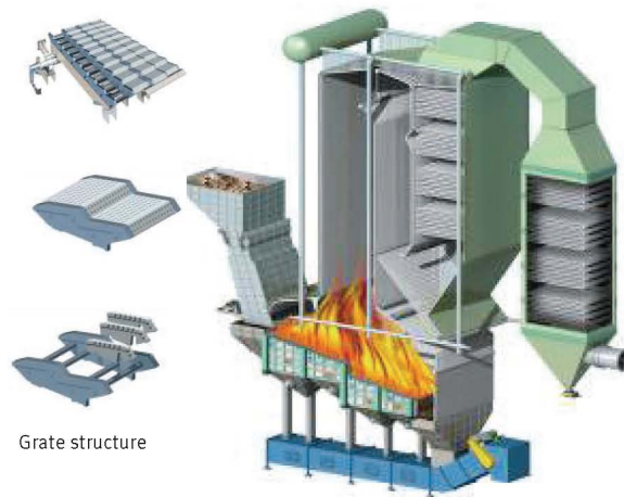
Stoker
